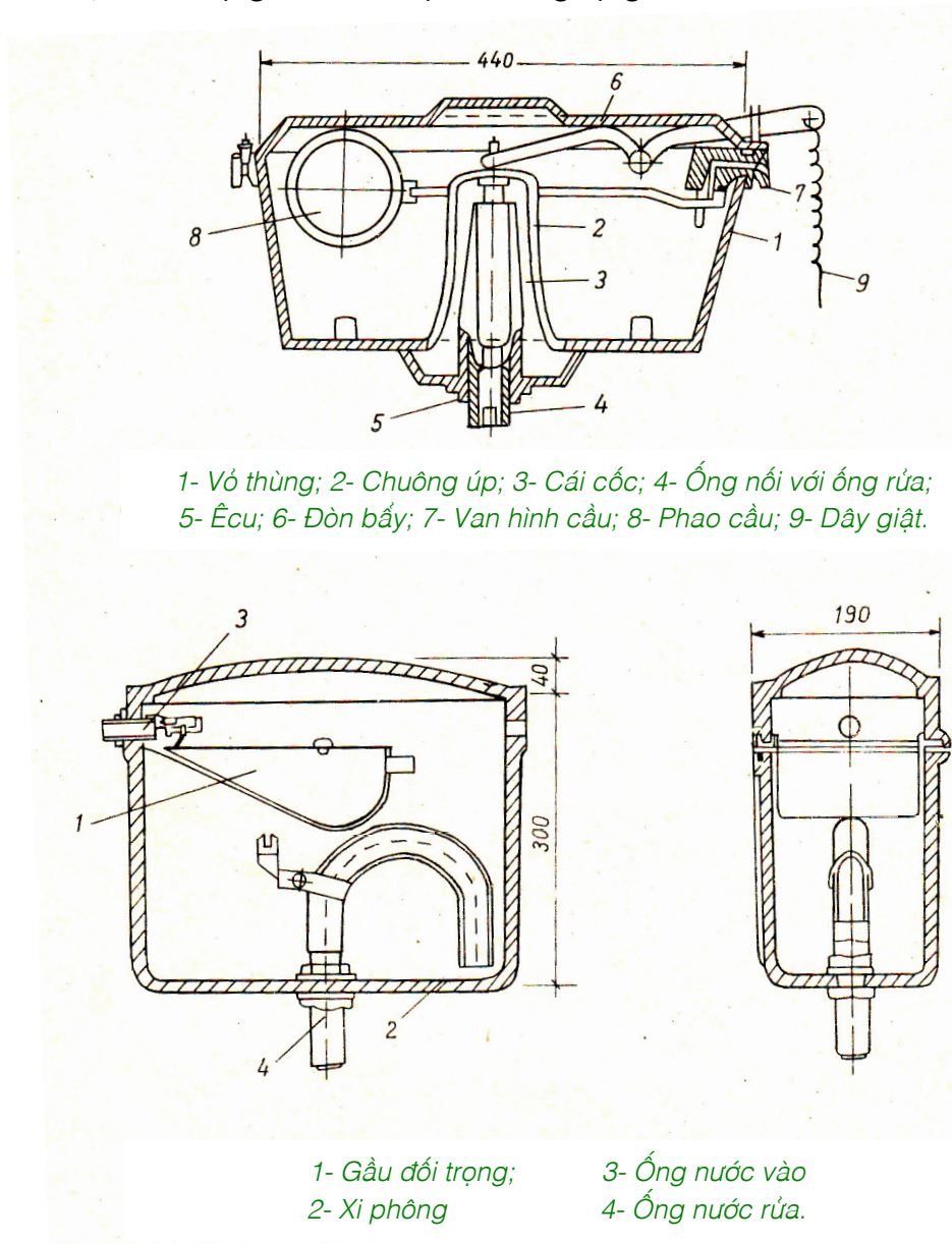
Hình 8.4: Cấu tạo thùng rửa xí.
