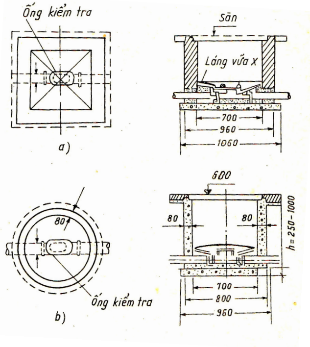
Hình 8.13: Giếng kiểm tra
