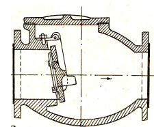
Hình 6.5: Van 1 chiều.
