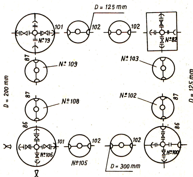
Hình 6.7: Chi tiết mạng lưới cấp nước.
