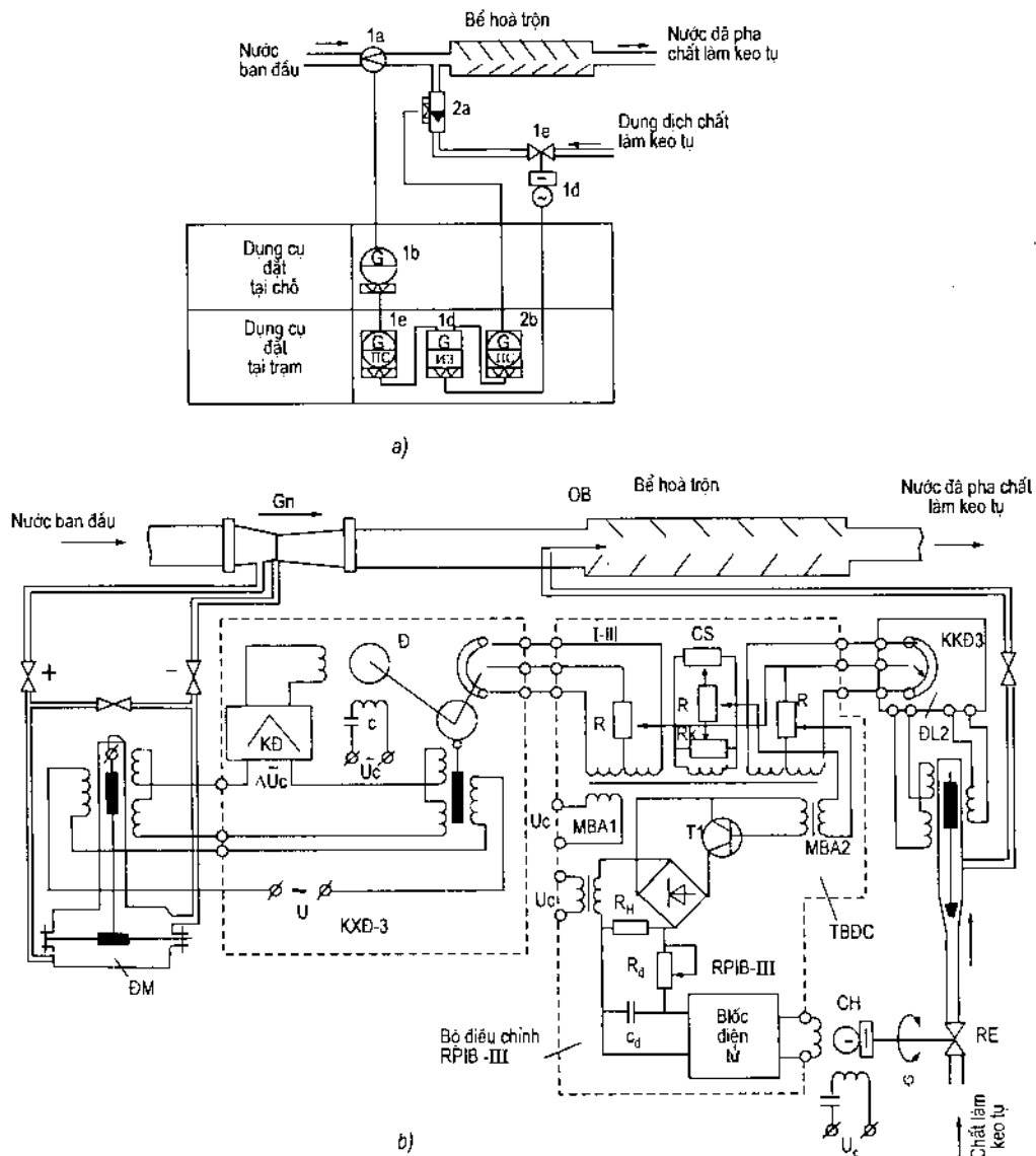
Hình 6-8: Sơ đồ điều tiết chất phản ứng tỉ lệ với lưu lượng nước cần xử lý
