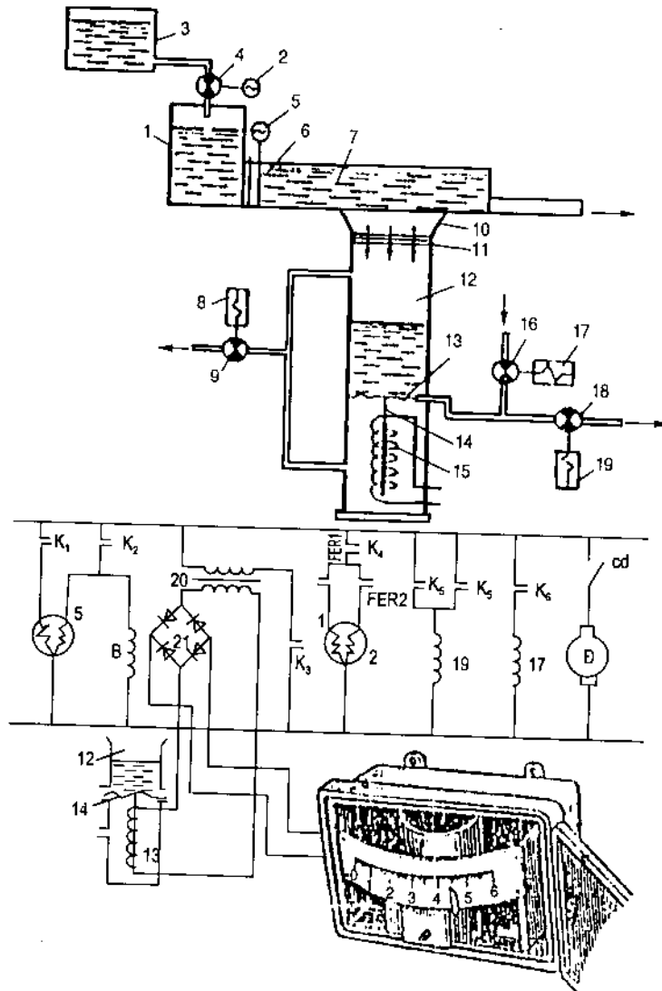
Hình 7-11: Sơ đồ điều tiết tự động chất phản ứng khi tách nước khỏi cặn bằng bể lọc chân không
