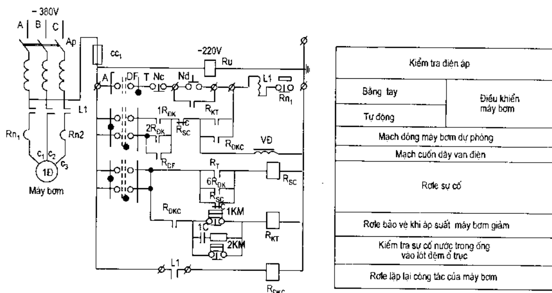
Hình 5-14: Sơ đồ điều khiển từng hệ thống máy bơm
