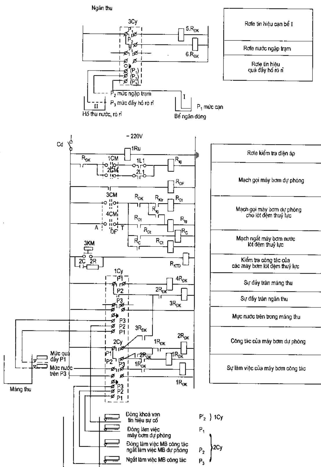
Hình 5-15: Sơ đồ mạch điện điều khiển chung cho các máy bơm trong trạm
