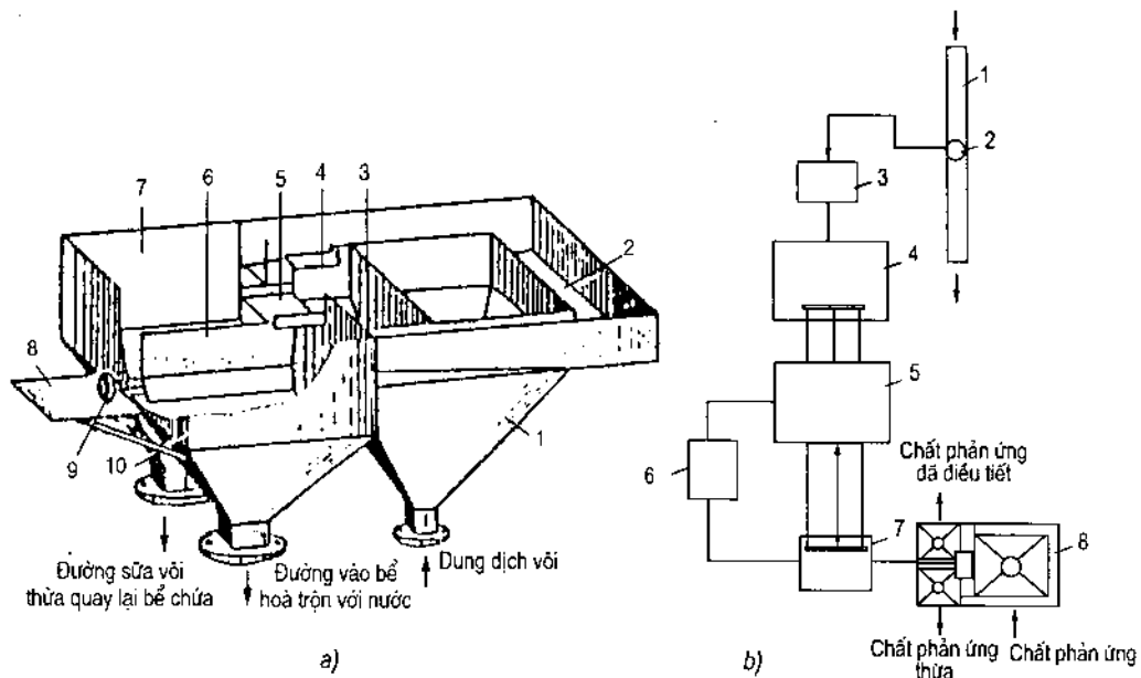
Hình 6-11: Thiết bị chuyên dụng điều tiết với sữa
